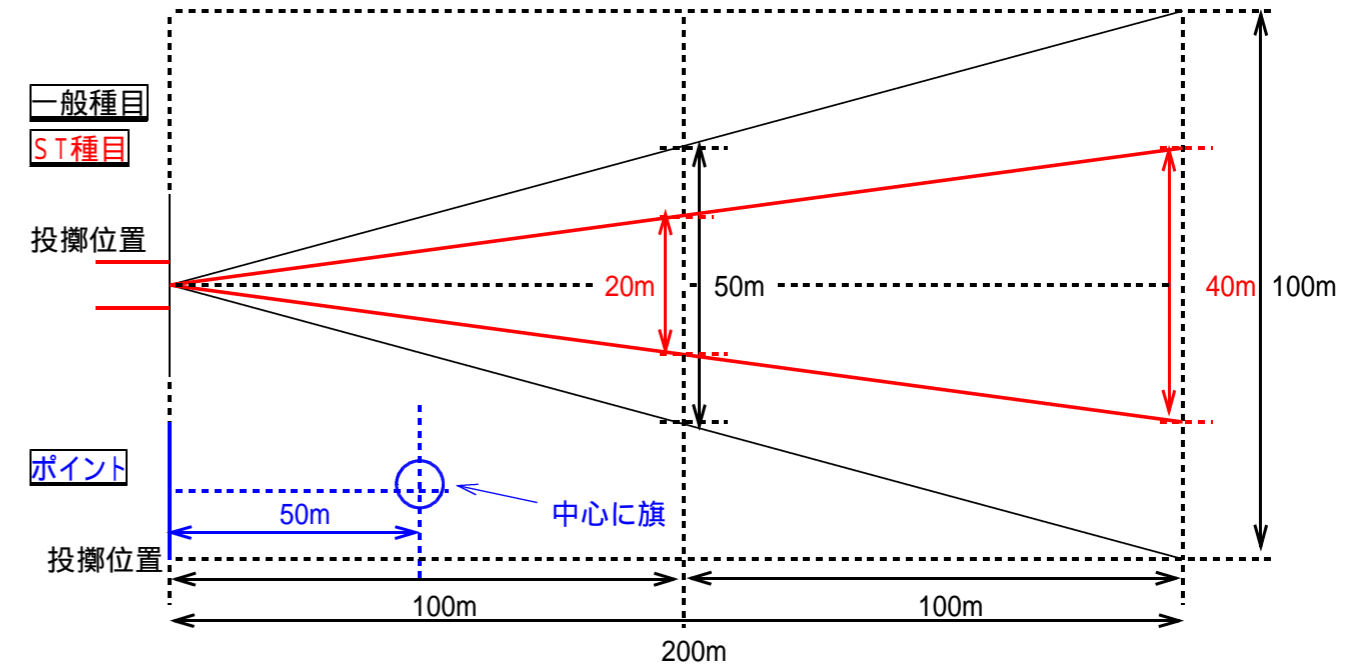
コート図
